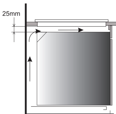
Vstavanie skrinky v pracovnej doske.
